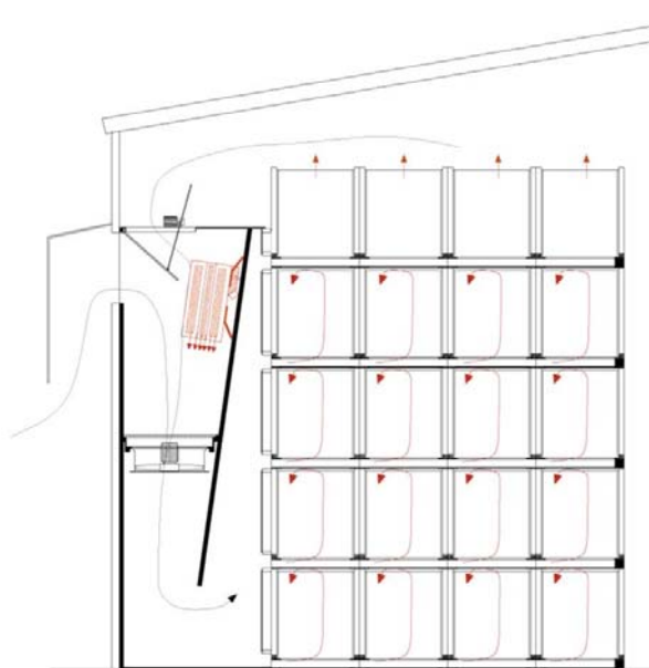
Luchtverdeling per kistlaag. Opwarming middels gasbrander of CV radiator.
