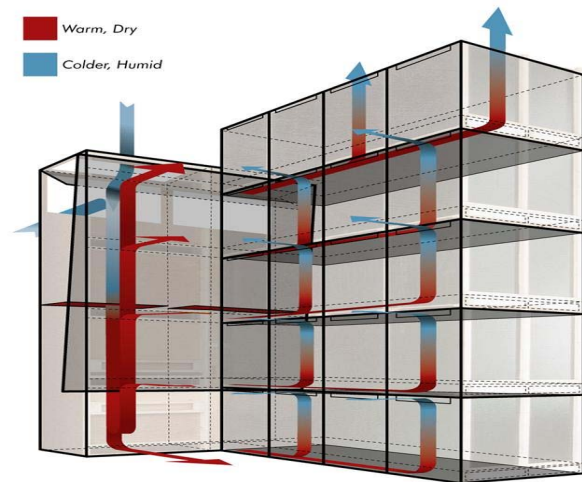
Drogen van zaad per kistlaag gescheiden. Aanzuigen buiten of binnenlucht.
